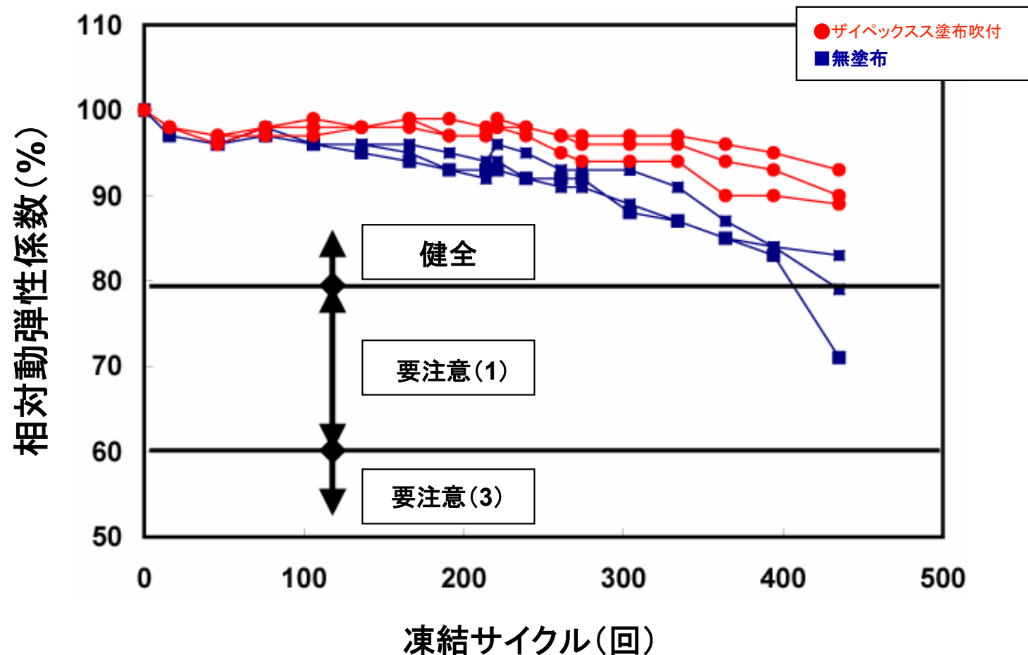
コンクリートの凍結融解試験
