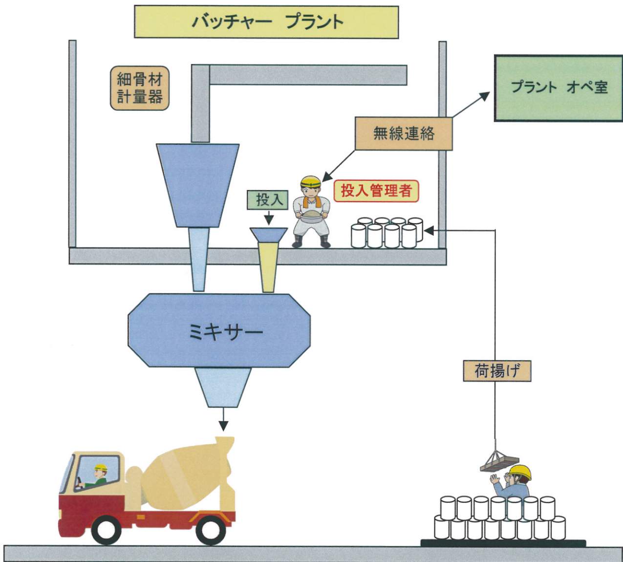
図-1 : 投入方法(混和材投入口より)
